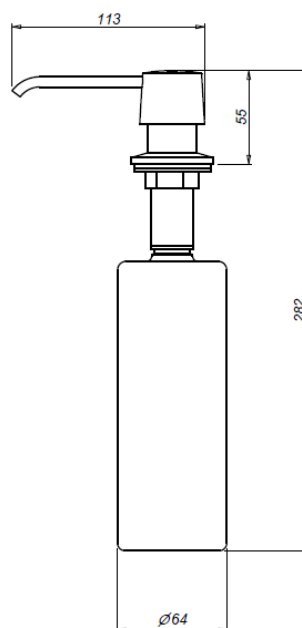
Desenho Técnico
